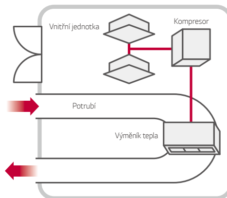
Případ připojení potrubím
