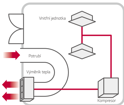
Případ přímého vstup/výstup
